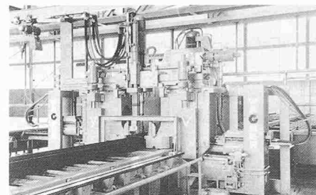
Bild 5. NC-gesteuertes Maschinenzentrum zum Bohren und Sägen
