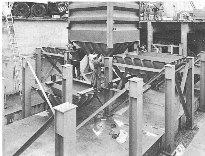
Bild 9. Der Aufbau dieser Siloanlage verlangt hohe Präzision beim Herstellen, Versetzen und Ausrichten
