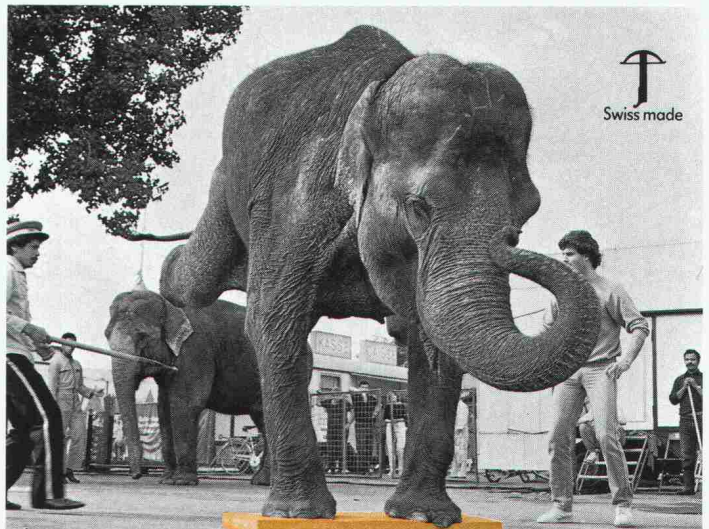
Der Elefant Tima des Zirkus Knie beim Druckfestigkeitstest mit der neuen Dämmplatte LURO HDF.
