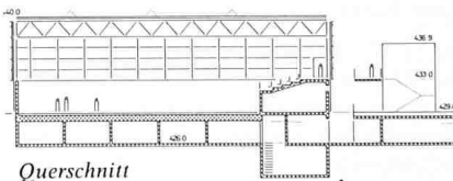
Querschnitt
