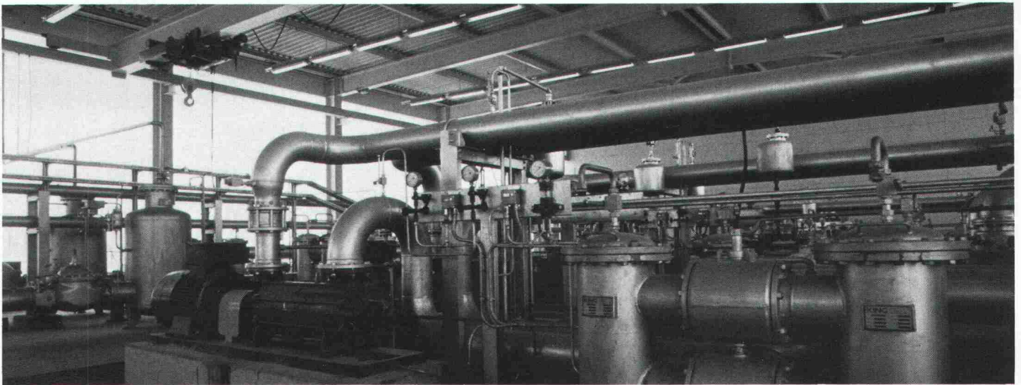
Brennstoff-Einlagerungspumpstation
