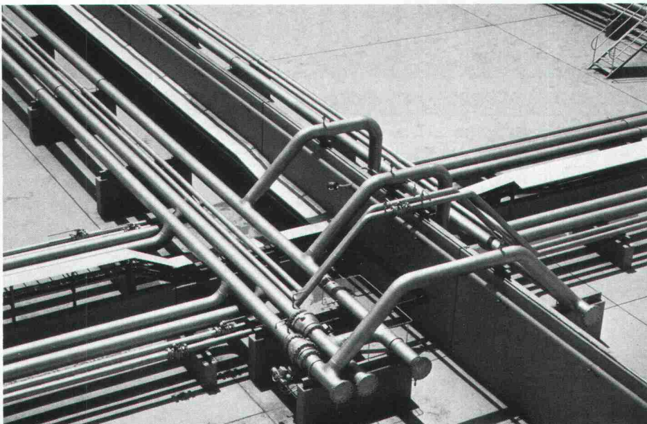
Brennstoff-Verteilnetz im Tankfeld
