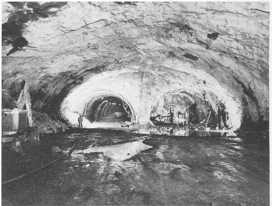
Bild 2. Kalottenausbruch in der Verzweigung. Links Haupttunnel Richtung Luzern mit Stahleinbau zur Sicherung des Mittelpfeilers, rechts Beginn des Ausbruchs im Anschlusstunnel
