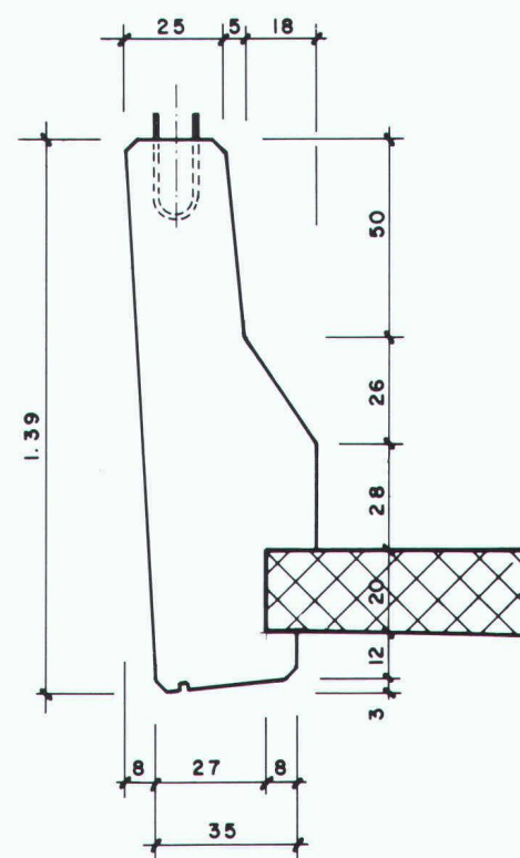
Bild 3: Querschnitt durch die Brüstung Typ «New Jersey» der Lorzentobelbrücke.
