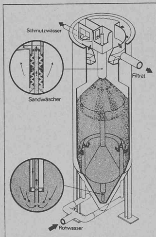
DynaSand-Filter (Schnitt)
