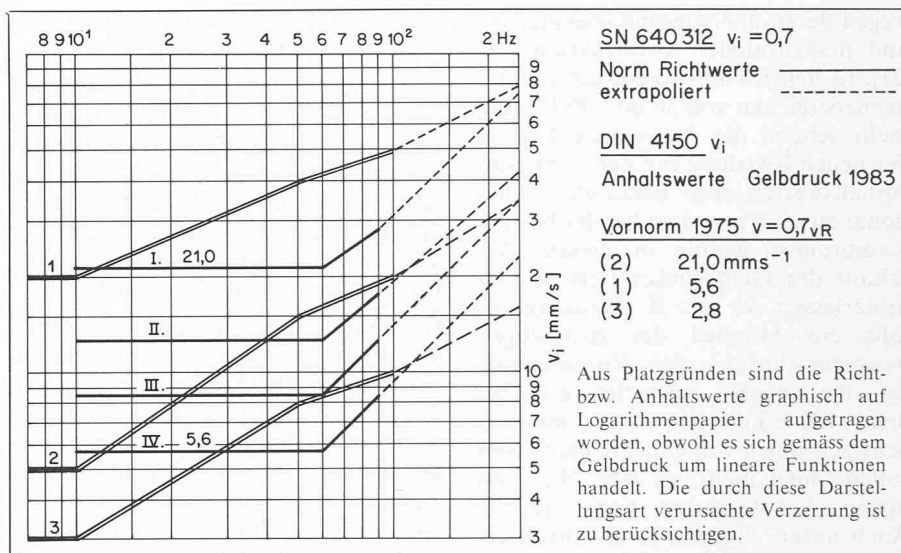
Bild 1. v_r -Werte [mm/s]. Einzelkomponente der Schwinggeschwindigkeit
