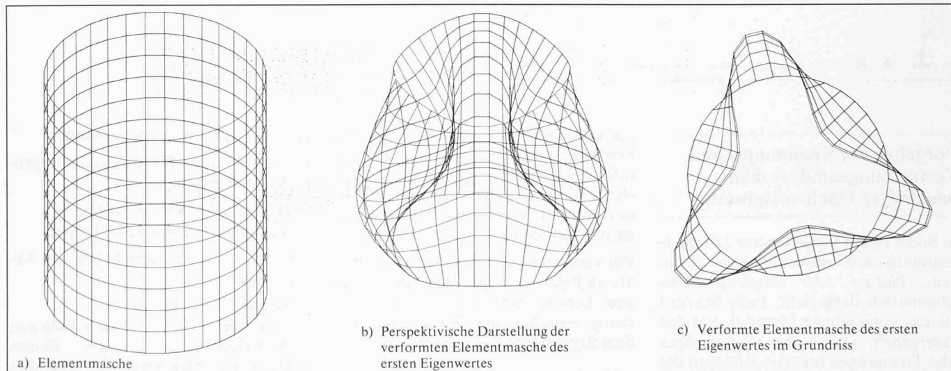
Bild 7. Elementmaschen der Finiten Element Berechnung des Kreiszyklinders
