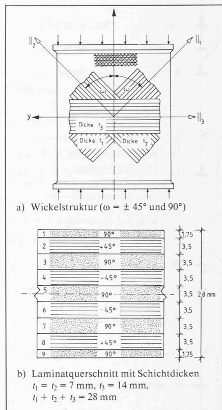
Bild 6. Aufbau der Kreiszyklinder
