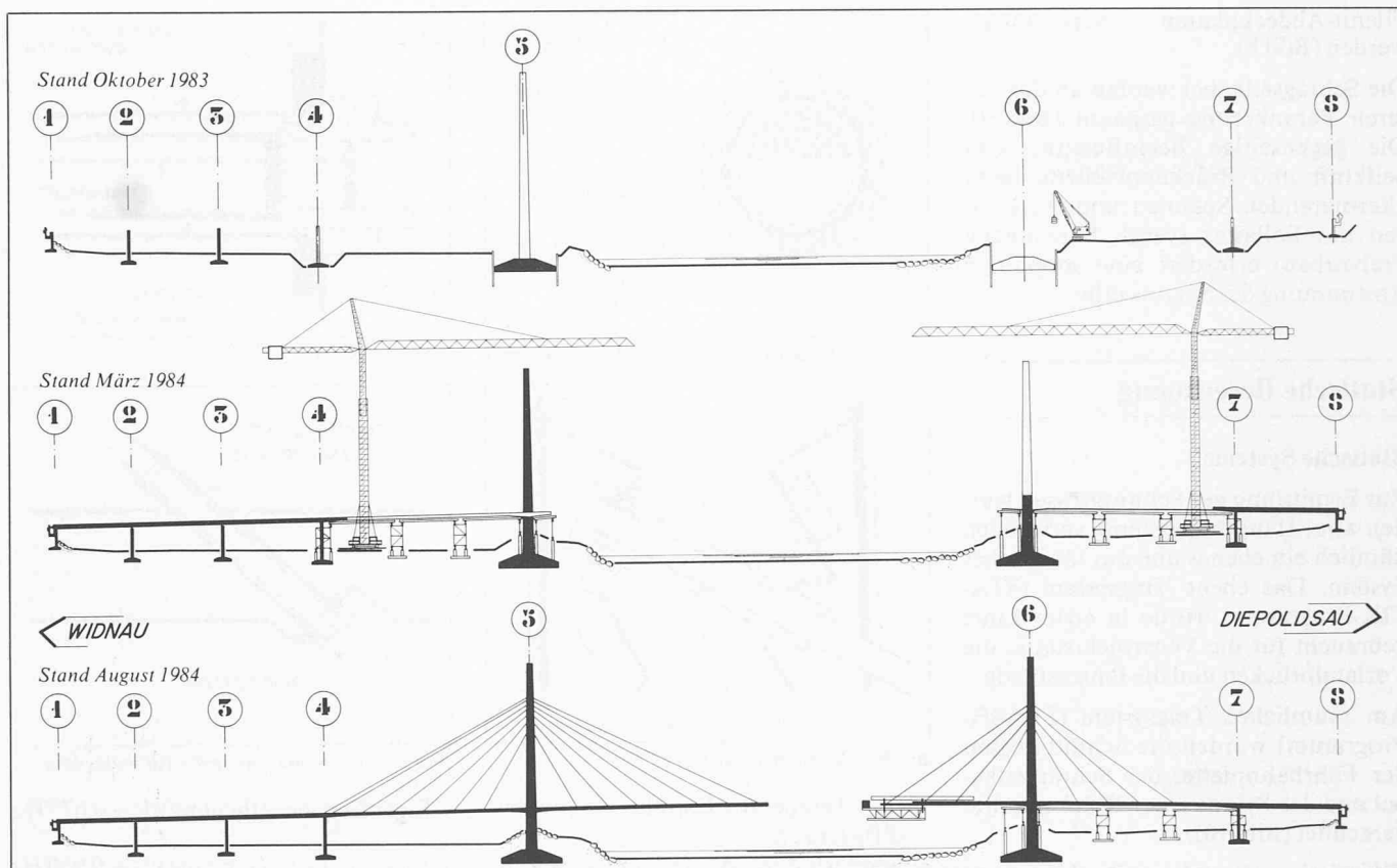
Bild 11. Bauphasenplan
