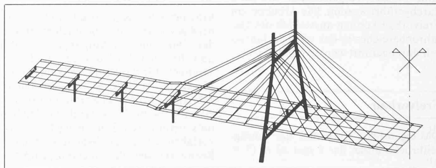
Bild 10. Räumliches Tragsystem
