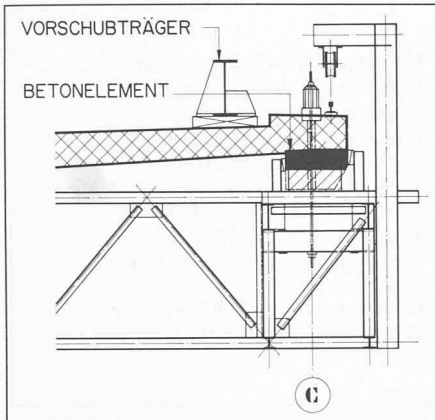
Bild 14. Vorbauwagen, Teilquerschnitt
