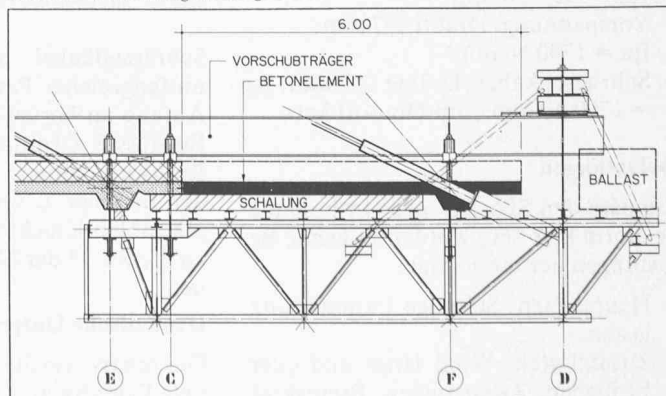
Bild 13. Vorbauwagen, Längsschnitt
