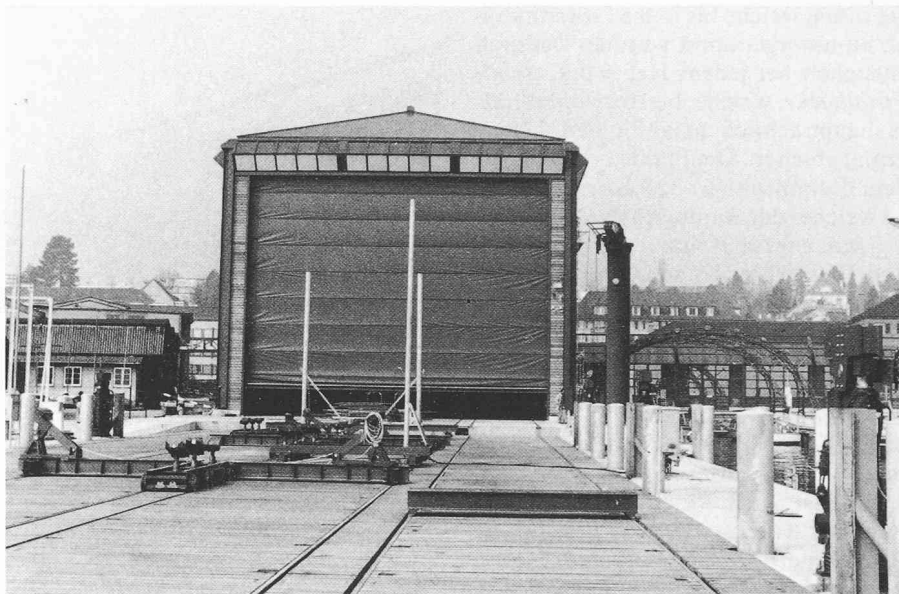
Bild 9. Blick von der Schiffsliift-Plattform gegen die geschlossene Werfthalle. Rechts erkennbar: ein Schiffsliiftsteg, Prellpfähle, Hubwerke und der Hafenkran
