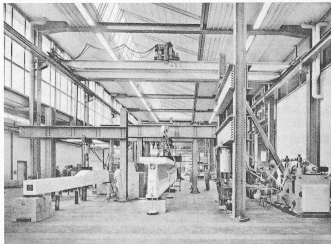
Neubau EMPA Dübendorf (1965). Aufspannboden
