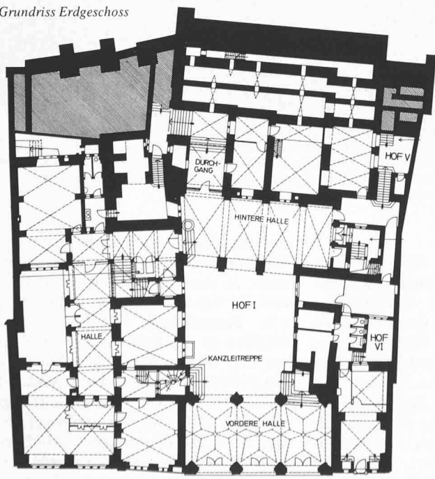
Rathaus Basel. Grundrisse und Schnitt, heutiger Bestand
