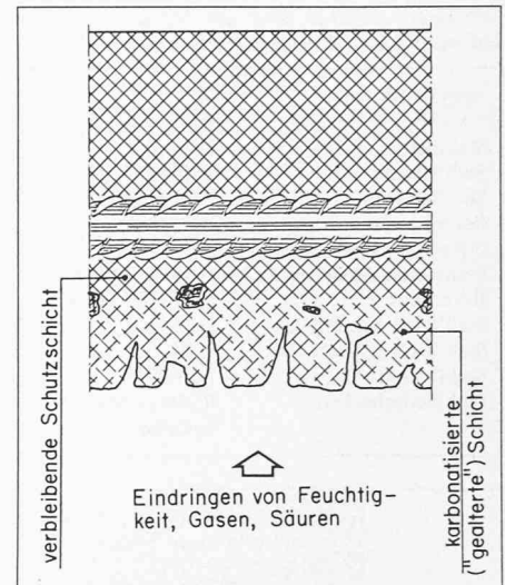
Bild 1. Karbonatisierte Zone innerhalb der Betondeckung
