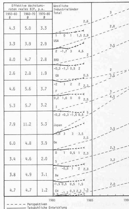
Bild 2. Kurz- und langfristige Perspektiven für einige westliche Industrieländer
