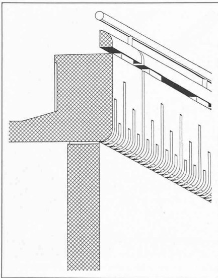
Bild 6. Künstlerische Gestaltung der 2,00 m hohen Überbauungsflächen der Tröglebrücke von Bild 4
