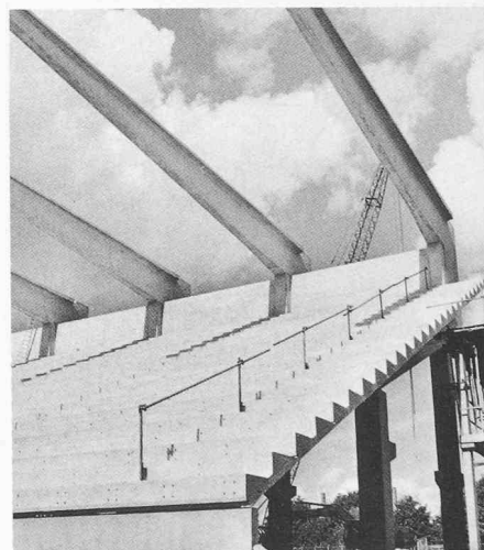
Bild 3. In nur 6 Monaten wurde die 16 m hohe Tribüne von Bild 2 aus 1730 Stahlbeton- und Spannbetonfertigteilen erstellt
