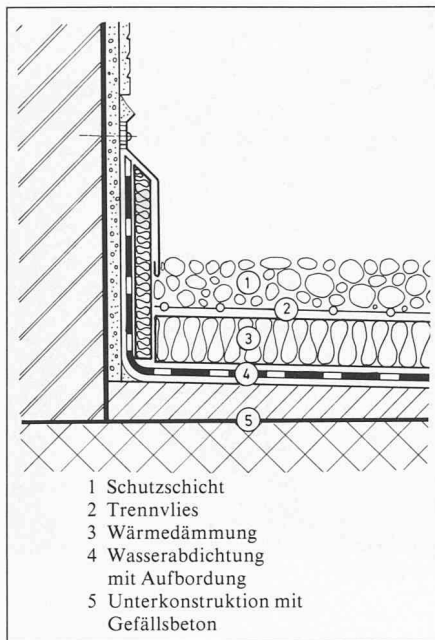
Bild 5. Umkehrdach und Aufbaurichtung der Abdichtung mit PBD
