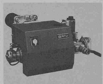
Brenner OE-2 Zweistoff, mit Haube und Regelstrecke
