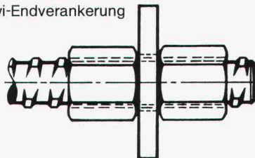
Gewi-Endverankerung
