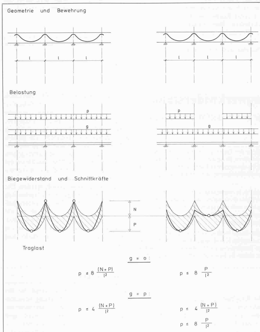
Bild 1. Durchlaufender Spannbetonträger
