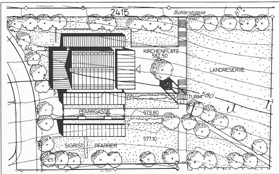
Lageplan 1: 1000
