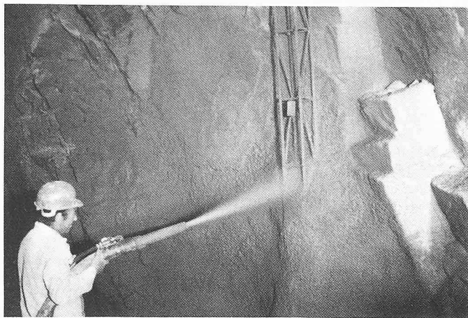
Bild 6. Einspritzen eines Gitterträgers im Versuchsstollen der Hagerbach AG; die Zugabe von Staubbinder unterdrückte die Staubentwicklung und erlaubte, mit \frac{1}{16} s Belichtungszeit zu fotografieren
