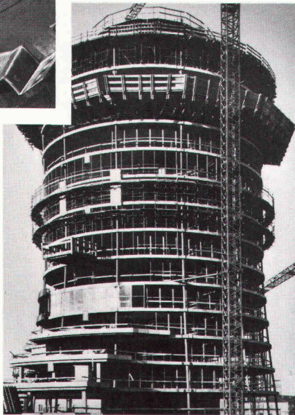
200 Vollstahlstützen für die BIZ
