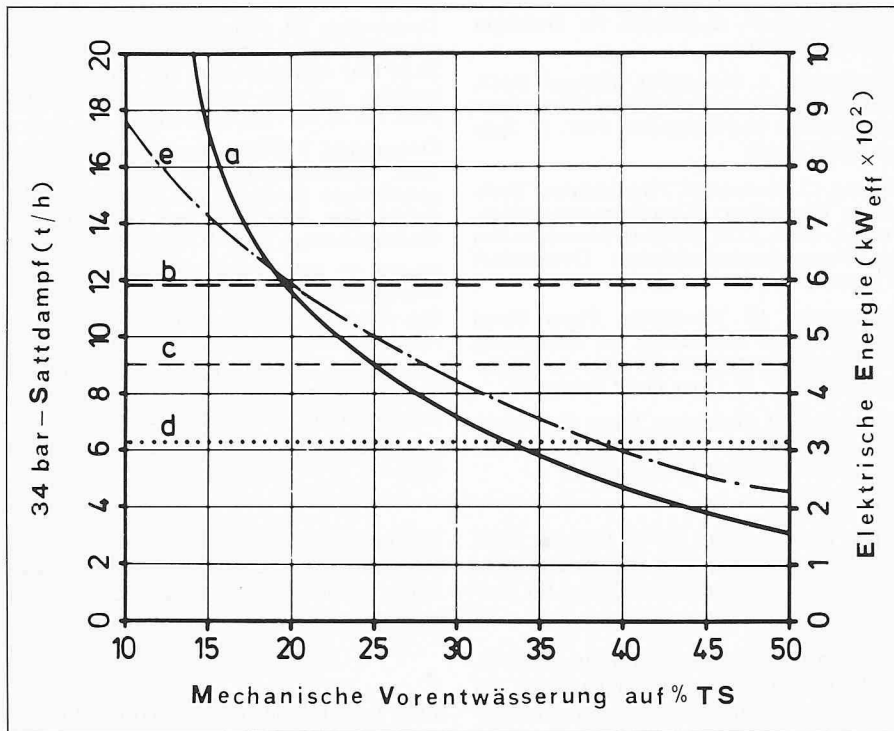
Beispiel für die Betriebswerte einer Klärschlamm-Verbrennungsanlage für 360 000 EGW. a: Sattdampfbedarf für die Trocknung. b-d: Sattdampfverzeugung bei der Verbrennung mit 12 500 kJ/kg unterem Heizwert (b), 9500 kJ/kg (c), 6700 kJ/kg (d). e: elektrischer Energiebedarf für Trocknung und Verbrennung.
