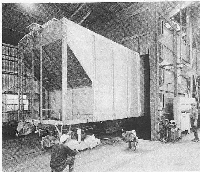
Bild 3. Amerikanischer Güterwagen von 21,3 m Länge beim Einfahren in eine mit 20 Schleuderrädern bestückte Gross-Strahlanlage in den Werken der Shippers Car Line Division der A.C.F. Industries Inc. in Longview, Texas. Man beachte den bauchigen Vorbau an den Stirnwänden sowie den Transportschemel in Spezialausführung mit Schutzabdeckungen aus verschleissfestem Material. Auch die automatische Kupplung ist zum Schutz vor der Wucht der Schleuderstrahlen mit dicken Gummitüchern umwickelt.
