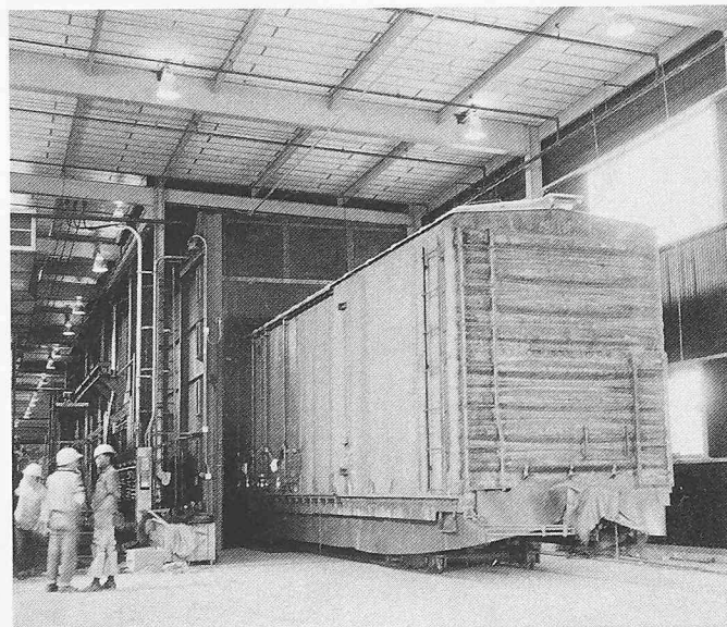
Bild 4. Amerikanischer Güterwagen von 18,3 m Länge beim Einfahren in eine mit 20 Schleuderrädern ausgerüstete Durchlaufstrahl-Anlage im Werk der American Car and Foundry Division of the A.C.F. Industries Inc. in St. Louis, Missouri, USA. Man beachte die gut sichtbaren Verwinkelungen an der Stirnwand des Wagens. Die automatische Kupplung und die Anschlusshähnen an der Stirnseite sind mit dicken Gummitüchern ange deckt.
