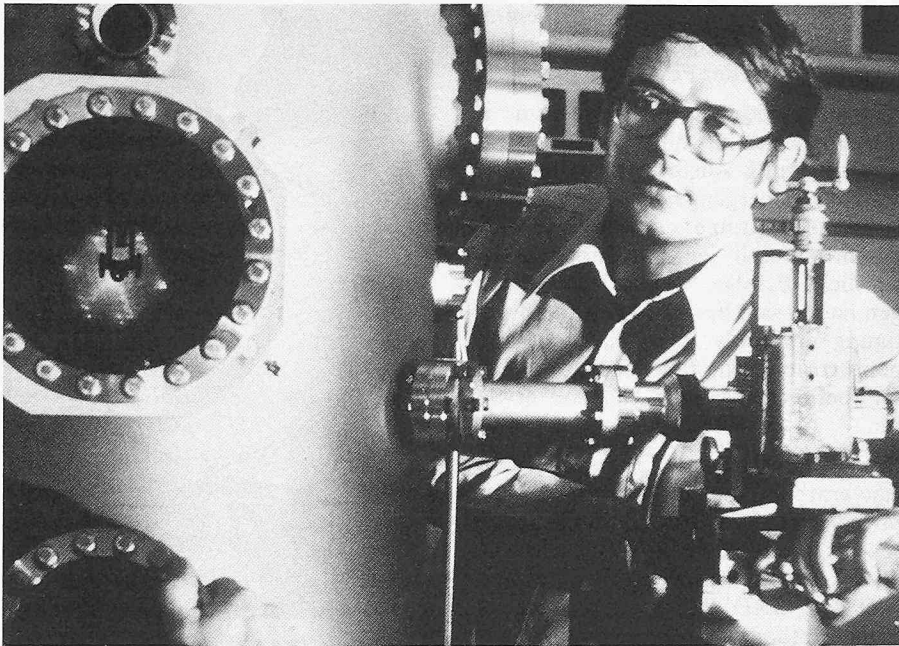
In Rüschlikon gebaute Hochvakuumkammer für Untersuchungen an Oberflächen. Bei idealen Bedingungen sind Prüfungen möglich mit Sekundärionen-Massenspektrometrie, Niederenergie-Elektronenbeugung, Auger- und Energieverlust-Elektronenspektroskopie sowie Atom- und Molekularstrahlstreuung bei thermischen Energien (TEAMS = Thermal Energy Atomic and Molecular Scattering) – Ende siebziger Jahre
