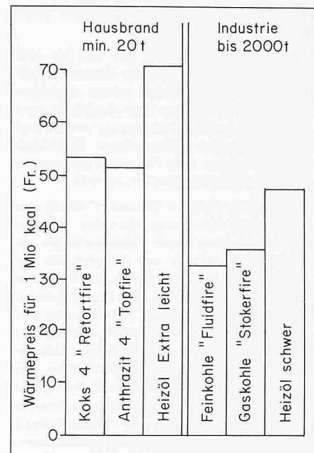
Bild 8. Durchschnittliche Wärmepreise für Verbraucher (Stand: 17. Aug. 1981).
