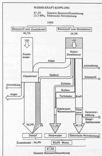
Energieflussdiagramm
