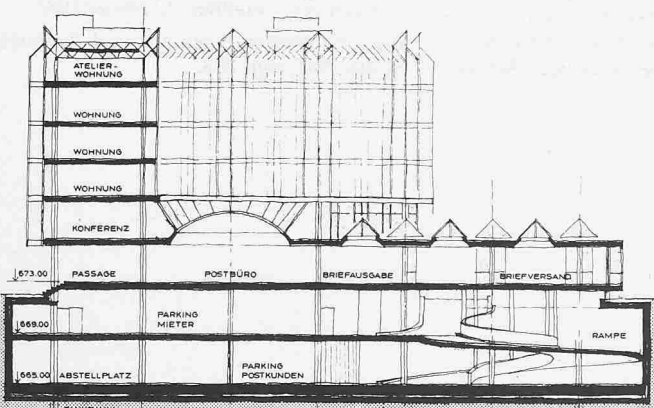
Schnitt 1:600
