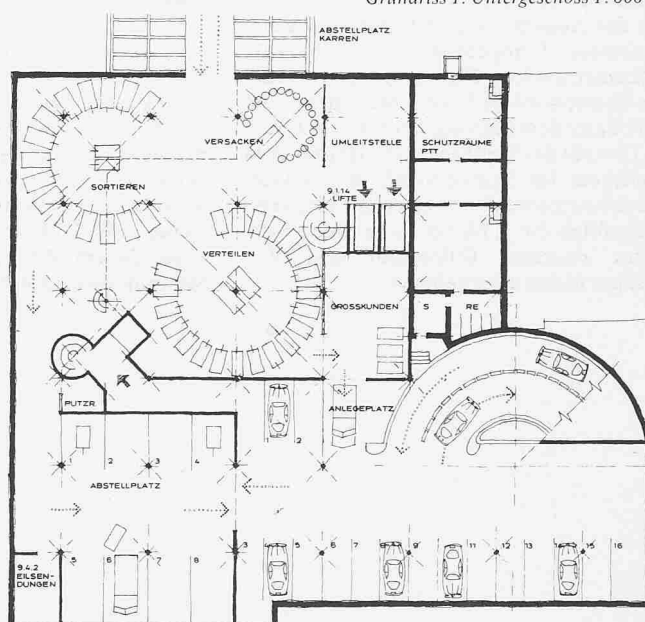
Grundriss 1. Untergeschoss 1:600
