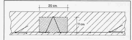
Bild 6. Querschnitt durch Armierung mit mitwirkender Betonfläche. Für die Aufnahme der Querkkräfte wird je Gitterträger eine mittragende Betonfläche von 11 \times 20 \text{ cm} gerechnet
