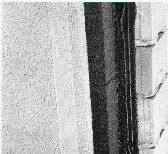
- Maueraufbau mit Permisol
