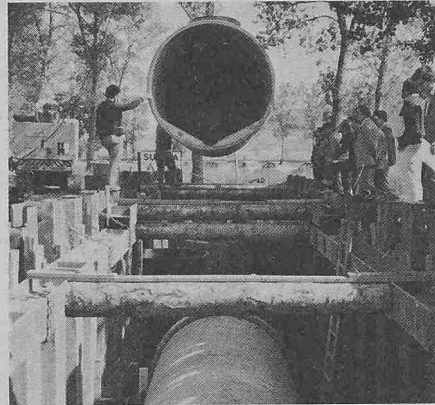
Die Elemente sind mit einer Druchlaufrinne, bestehend aus Drittelschalen und Eternitplatten, ausgestattet
