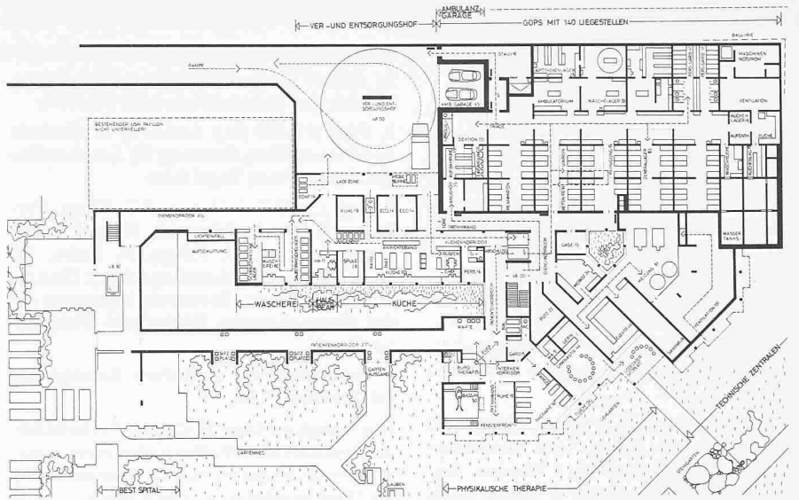
Grundriss 1. Untergeschoss 1:900
