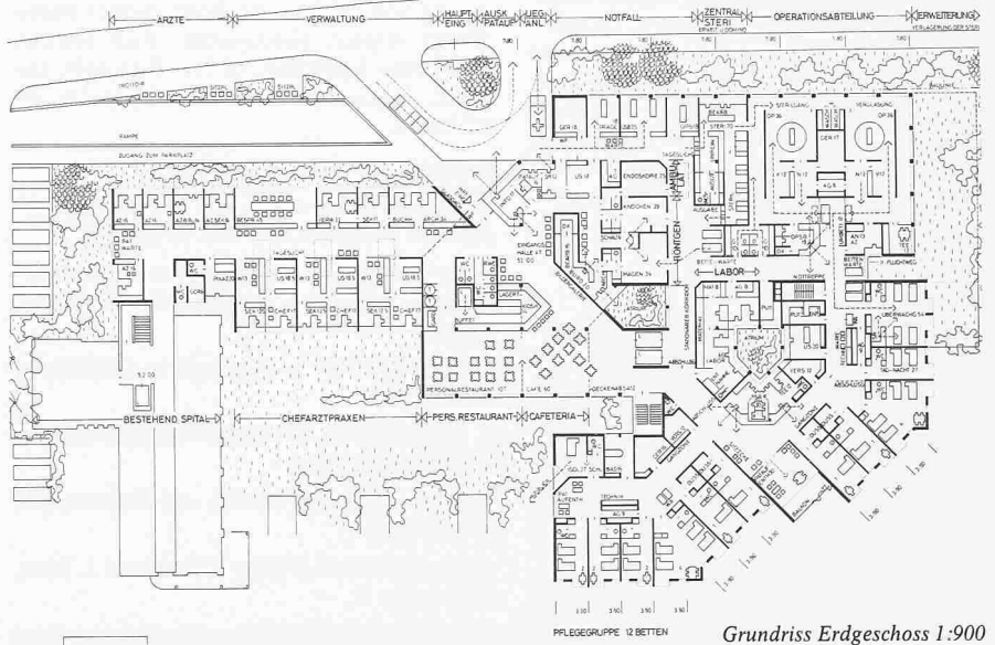
Grundriss Erdgeschoss 1:900
