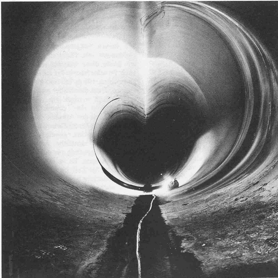
Bild 6. Eingebeulte Druckschachtpanzerung
