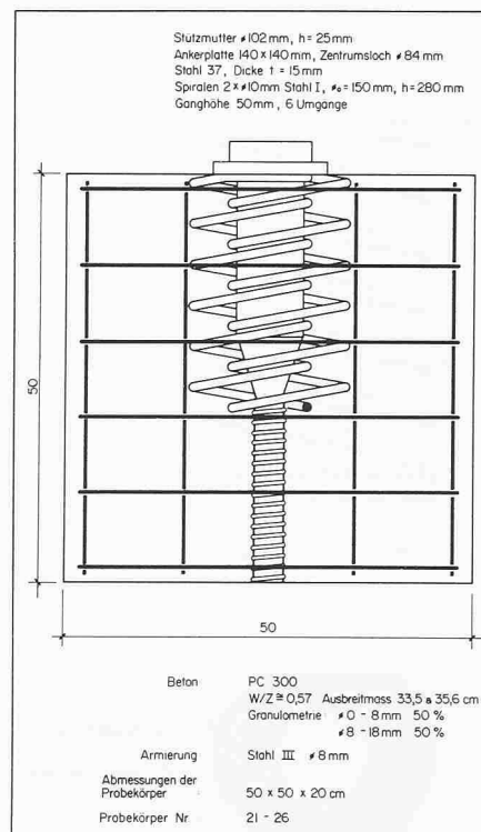
Bild 2. Aufbau der Probekörper mit variabler Plattenstärke zur Ermittlung des Einflusses der Plattensteifigkeit
