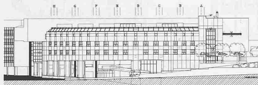
Ostfassade gegen Schulhausplatz und Altstadt
