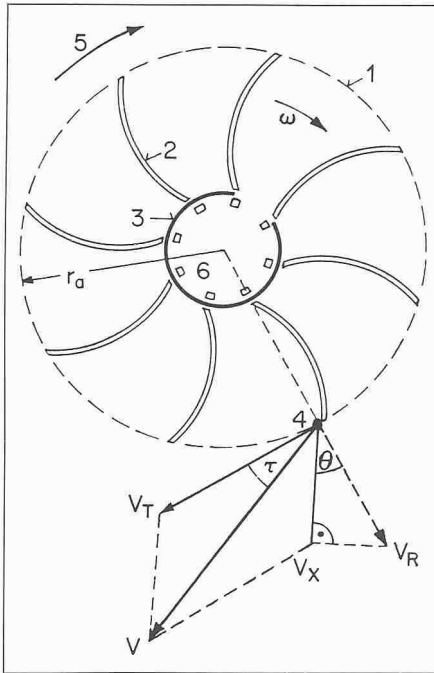
Bild 11. Geschwindigkeits-Diagramm in Vektor-Darstellung zur Berechnung der Abwurfgeschwindigkeit eines Strahlmittels beim Austritt aus einem mit nach vorn gleichförmig gekrümmten, konkaven Wurfschaufeln bestückten Schleuderrad.
