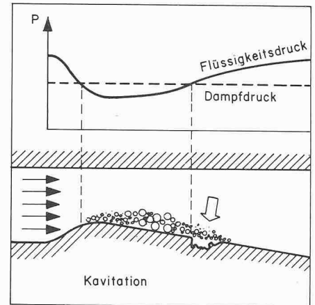
Bild 4. Prinzip der Strömungskavitation
