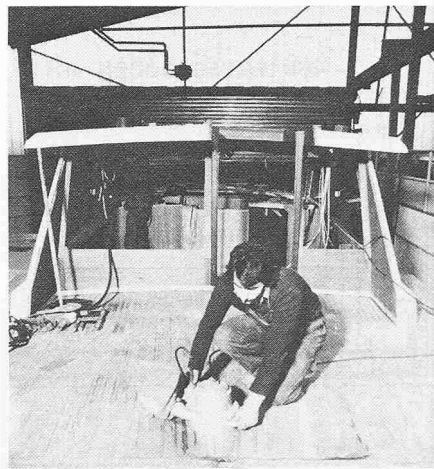
Die Fugen zwischen den Riemen eines hölzernen Decks einer Yacht wurden mit Polyurethan-Kunststoffkitt gedichtet. Anschliessend wurde die Deckfläche noch mit der Schleifscheibe bearbeitet. Trotz der harten Beanspruchung wurde der Kitt nicht aus den Fugen zwischen den Decksplanken herausgerissen und die Schleifscheibe wurde auch nicht verschmiert
