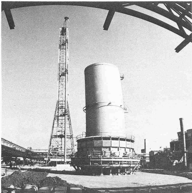
Fackelanlage, in der brennbare Gase gefahrlos und umweltfreundlich verbrannt werden können. Die Fackelanlage besteht aus einer Hochfackel (links), die sich von anderen Fackeln dieser Art nur durch ihre Höhe unterscheidet, und einer Bodenfackel (rechts), wie sie auf dem Werkgelände erstmalig errichtet wurde. Die Bodenfackel besteht im wesentlichen aus einem Zylinder von 10 m Durchmesser und einer Höhe von 27 m. Die Kapazität der Bodenfackel reicht aus, um die bei planmässigen Anfahr- und Abstellvorgängen anfallenden Gasmengen zu verbrennen; die Hochfackel spricht erst dann an, wenn – zum Beispiel beim Ausfall eines Verdichters – kurzfristig grössere Gasmengen verbrannt werden müssen
