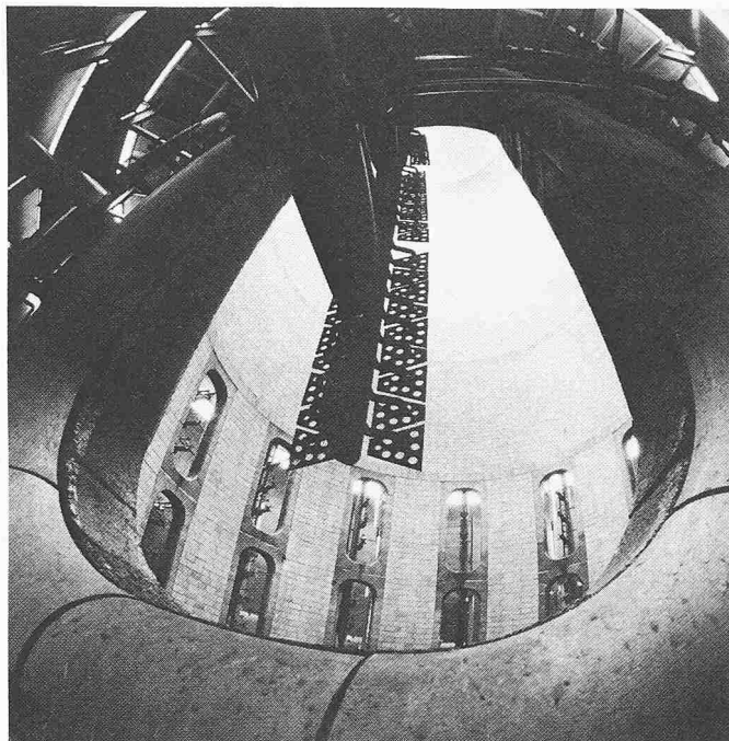
Blick in die Bodenfackel, in der die Flammen innerhalb eines Zylinders von 10 m Durchmesser und 27 m Höhe brennen und deshalb nicht direkt sichtbar sind; die Schallausbreitung ist ebenfalls erheblich gedämpft
