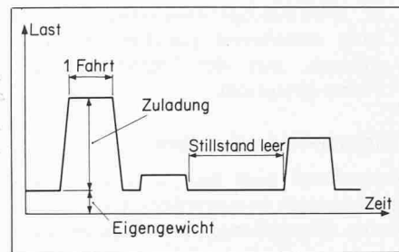
Bild 8. Grundlastschwankung infolge Be- und Entladens
