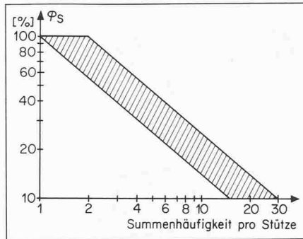
Bild 11. Aufretenshäufigkeit des Stossfaktors \phi_s je Stützenüberfahrt
