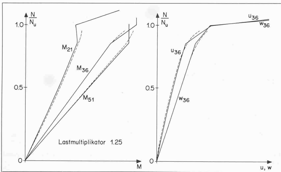
Bild 11. Quergefederter Rahmen mit \gamma_s = 1.7 ; Verlauf der Momente und der Auslenkungen nach der Fliessgelenktheorie 2. Ordnung
