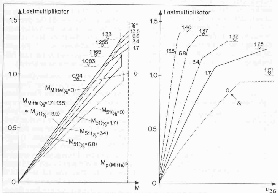
Bild 13. Quergefederter Rahmen mit verschiedenen Steifigkeitswerten \gamma_s ; Vergleich des Verlaufes der Momente und der Auslenkungen nach der Fliessgelenktheorie
