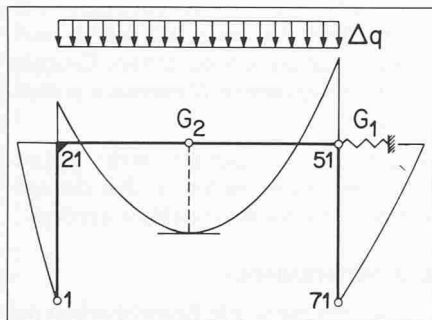
Bild 12. Quergefederter Rahmen mit \gamma_s = 1.7 ; Tragsystem nach der Bildung des zweiten Fliessgelenkes
