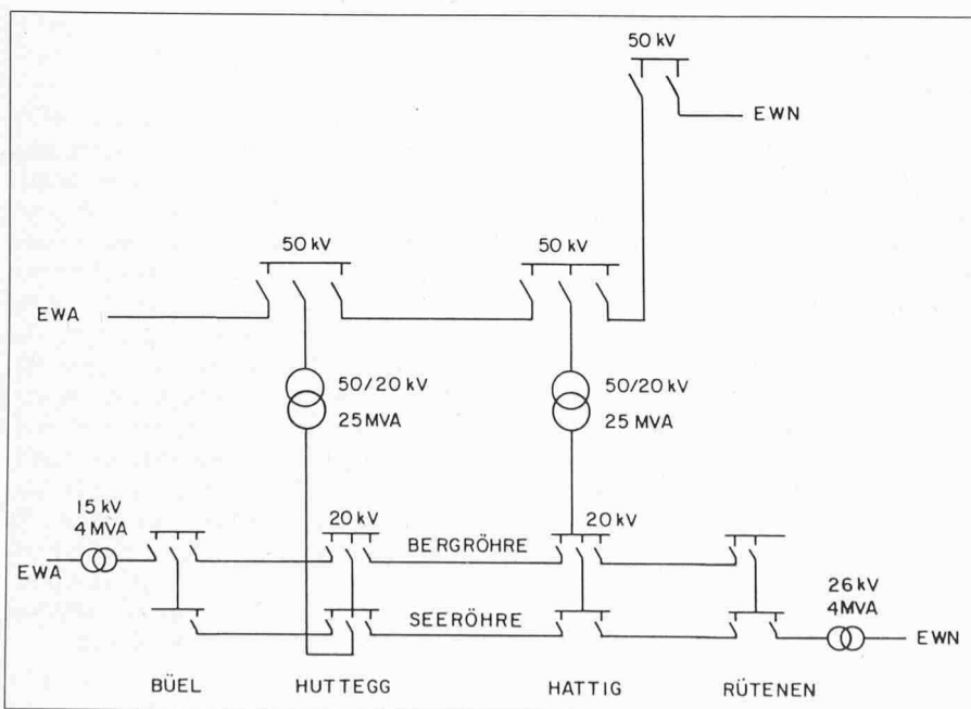
Bild 1. Übersicht Energieversorgung
