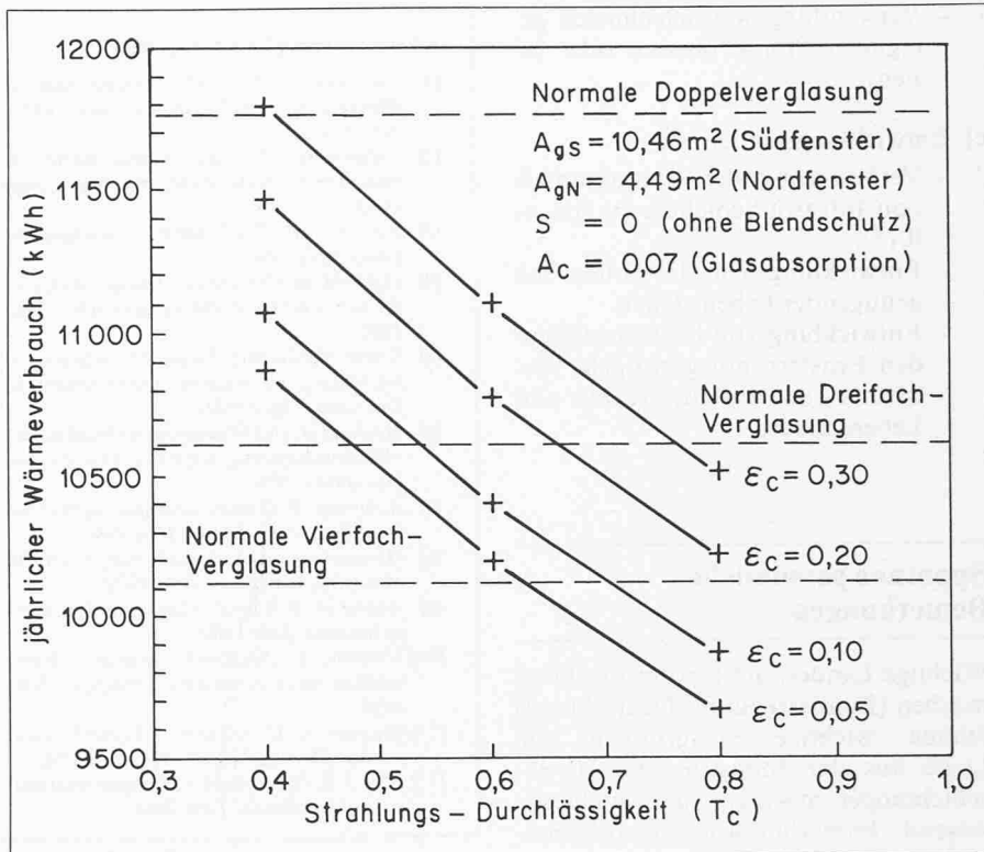
Bild 5. Jährlicher Raumheizungsbedarf eines Standard-Haustyps ( 147 \text{ m}^2 Wohnfläche) in Stockholm, Schweden, in Abhängigkeit von verschiedenen Durchlässigkeiten/Emissivitäten ( \epsilon_c ) der Glas-IR-Beschichtung (nach Adamson [9])
