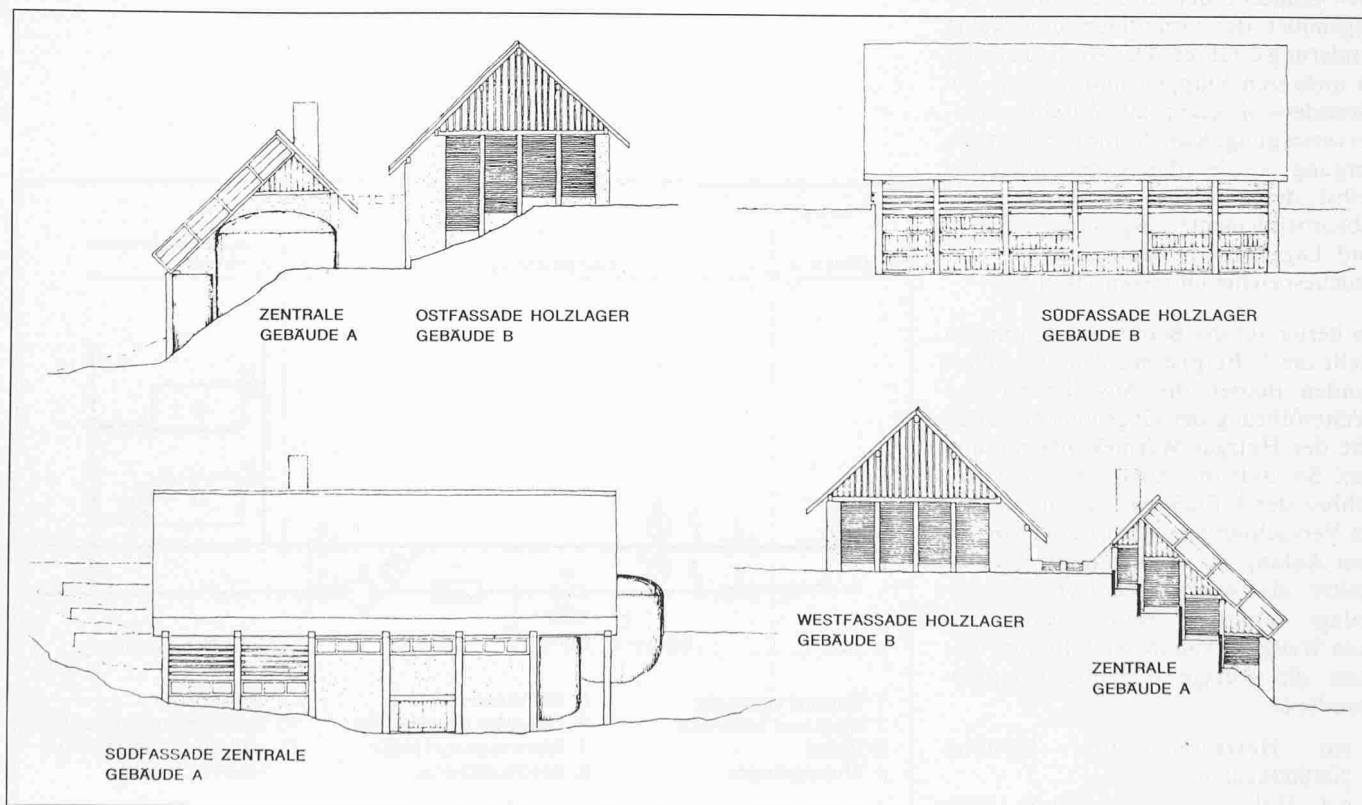
Bild 11. Gebäudefassaden
