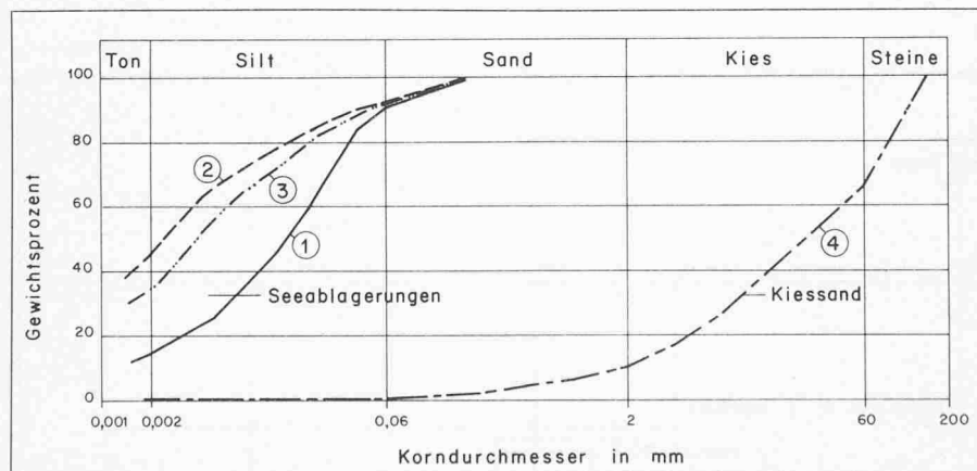
Bild 7. Kornverteilungen Seeablagerungen und Kiessand in Zürich. Probe 3 entspricht dem dem Scherversuch unterzogenen Material
