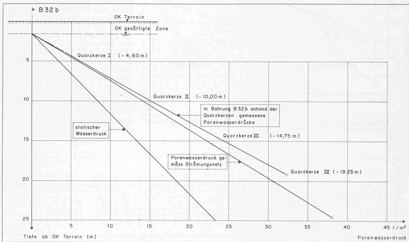
Bild 4. Darstellung der gemessenen Porenwasserspannungen in Gneida. Man beachte den linearen Druckabbau von Quarzkerze IV bis Quarzkerze I
