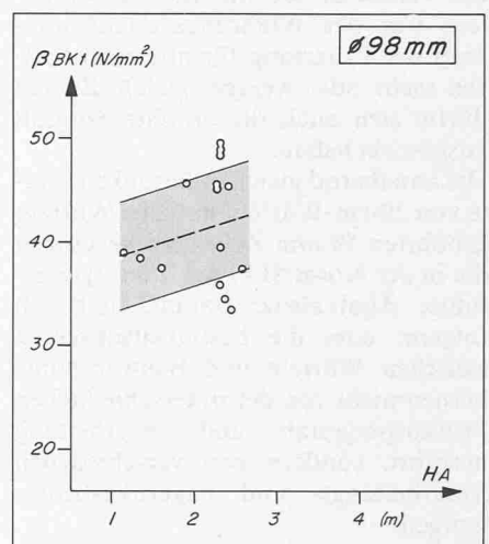
Diagramm 9. Bohrkernfestigkeit und Auflasthöhe (Wände)
