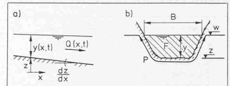
Bild 1. Skizze zur Definition der massgebenden Grössen für die Berechnung instationärer Abflüsse in offenen Gerinnen.
