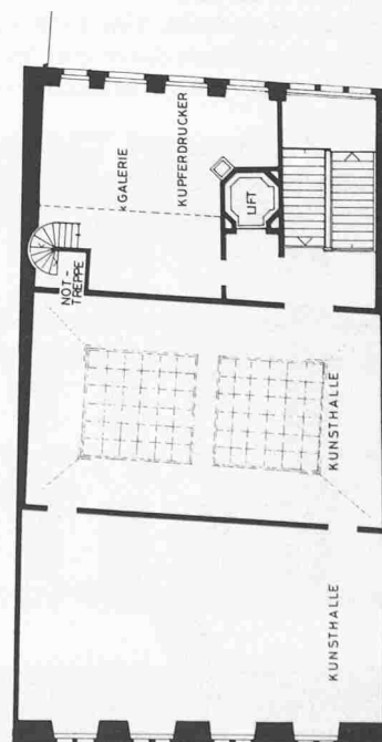
2. Obergeschoss 1:250
