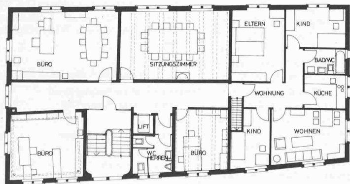
3. Obergeschoss 1:250
