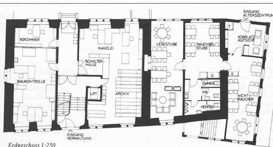
Erdgeschoss 1:250
