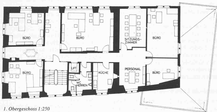
1. Obergeschoss 1:250
